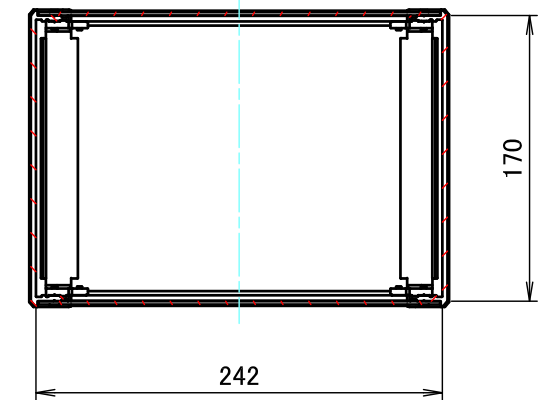
C-C ( 1:4.5 )
