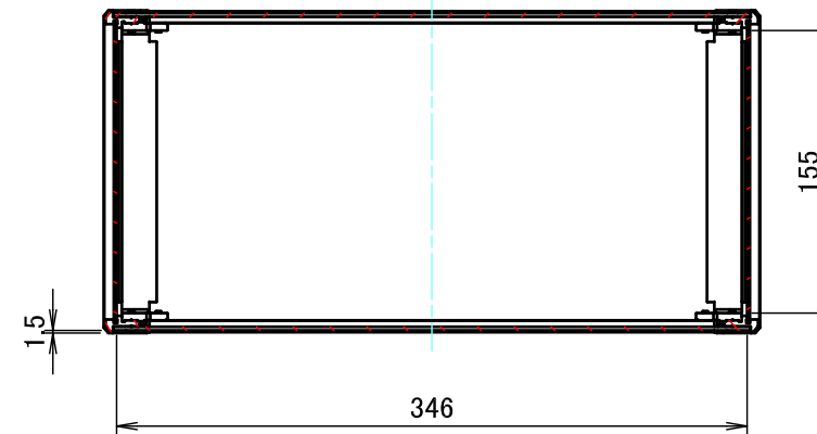
A-A ( 1:4.5 )
