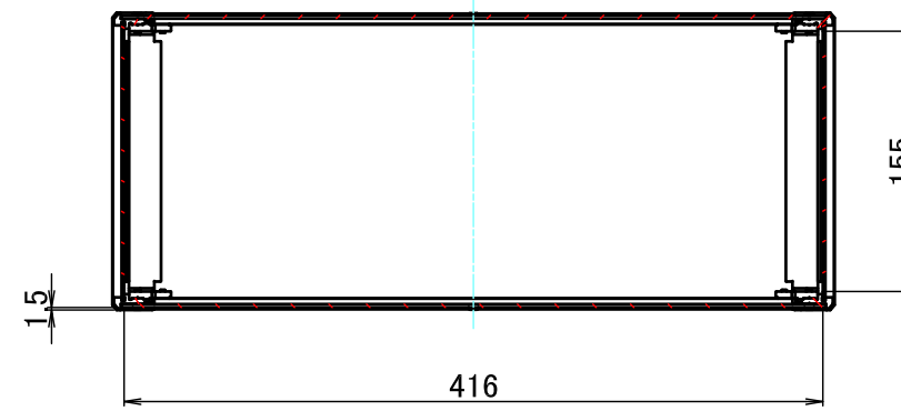
A-A (1:5)
