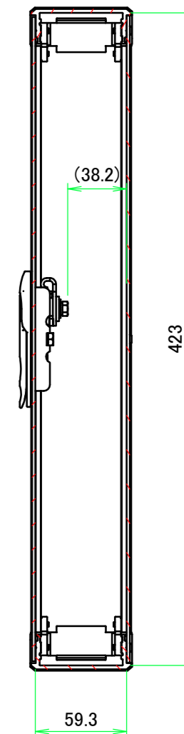
B-B (1:3.5)
