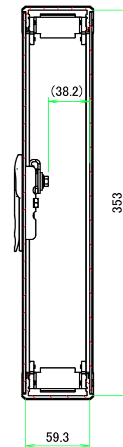
B-B (1:3.5)
