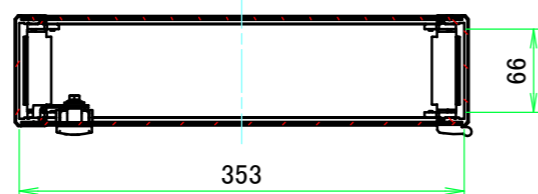
A-A (1:6)
