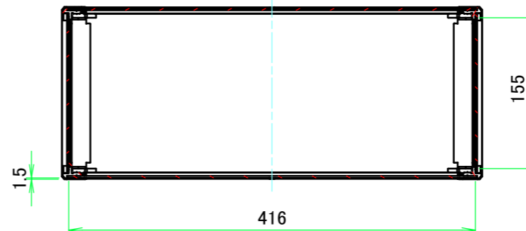
A-A ( 1 :5.5 )
