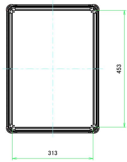
B-B (1 : 6.5)
