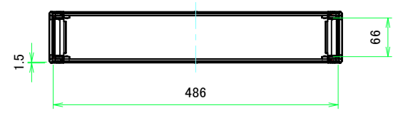
A-A (1 : 6.5)
