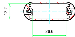
A-A (1:1)
