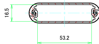
A-A (1:1.5)
