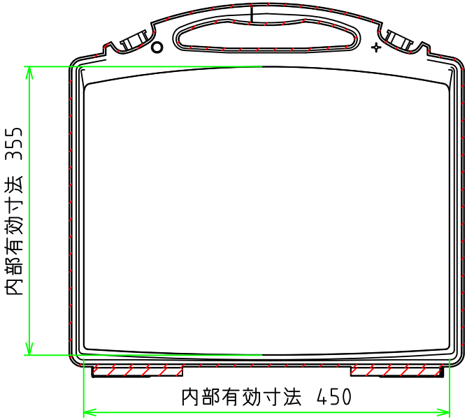
B-B 断面図
