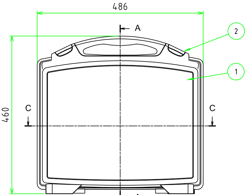
カバー側
